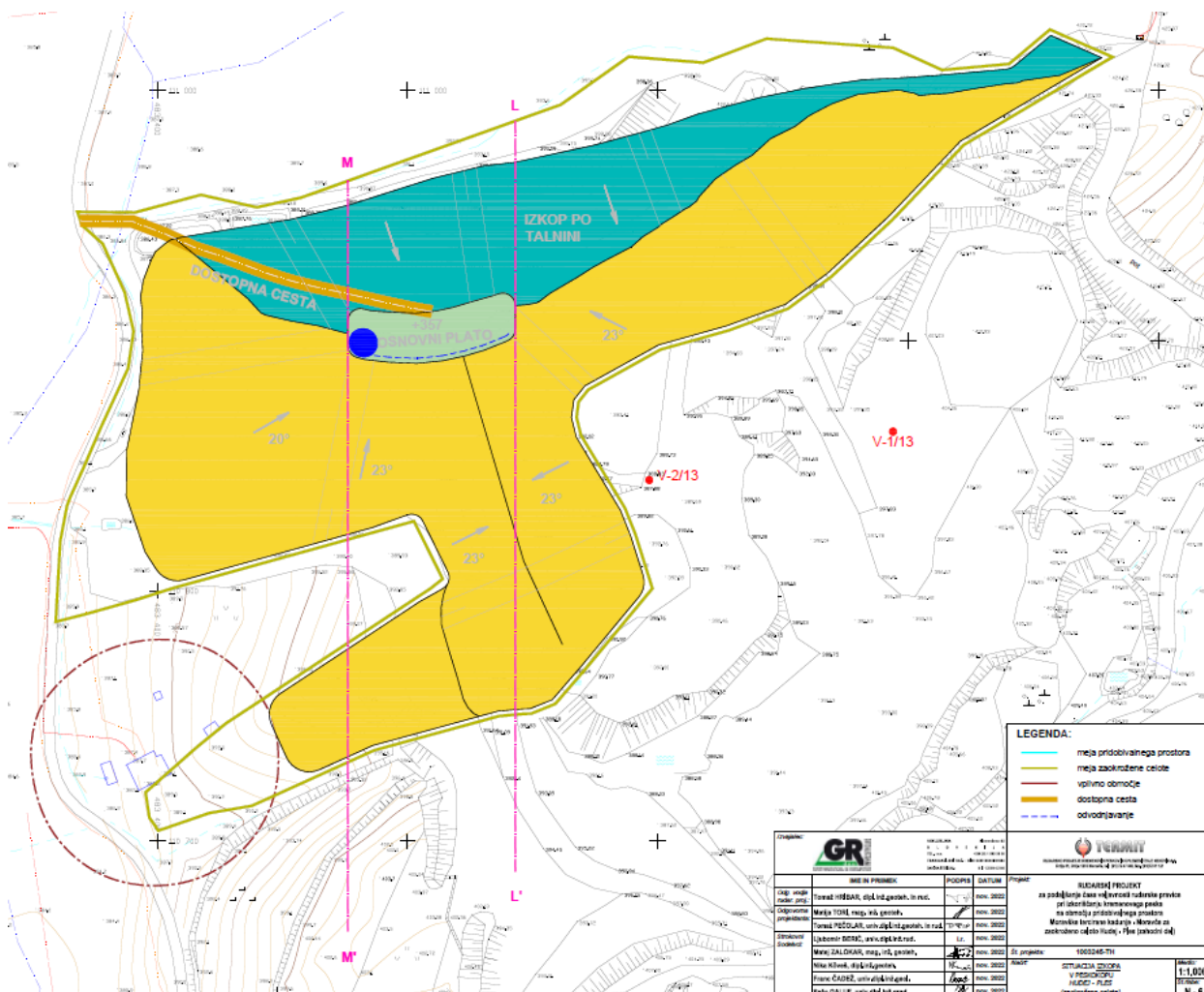
Slika 13: Situacija izkopa peskokopa Hudej-Ples (zahodni del) (vir: Rudarski projekt, 2022)
